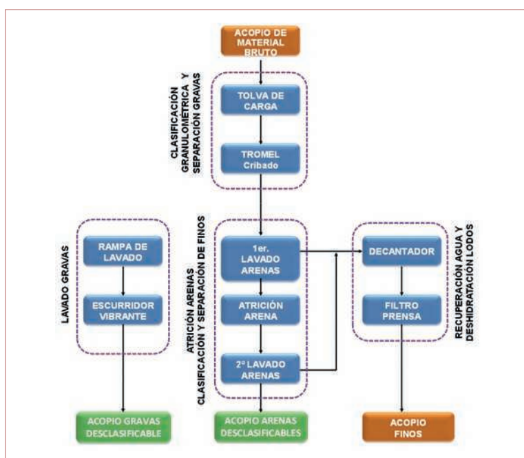
Esquema de las diferentes partes de proceso de tratamiento de las tierras, así como su destino final, según éstas sean tratadas en la planta de lavado de la central José Cabrera.
