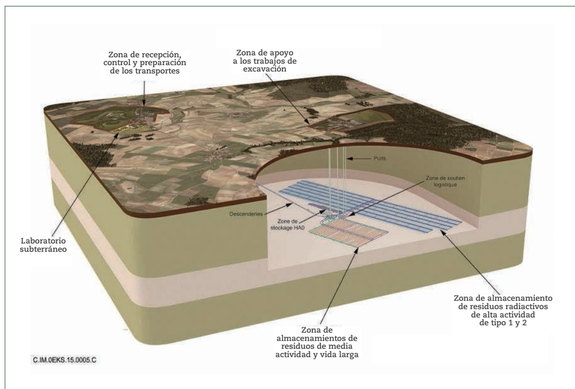
Diseño conceptual de las instalaciones de CIGEO.
