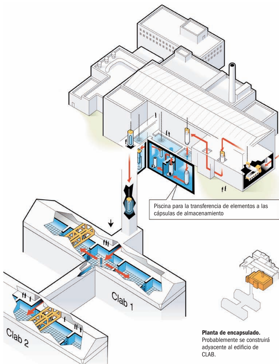
Esquema de los procesos que se llevan a cabo en las instalaciones CLAB.
